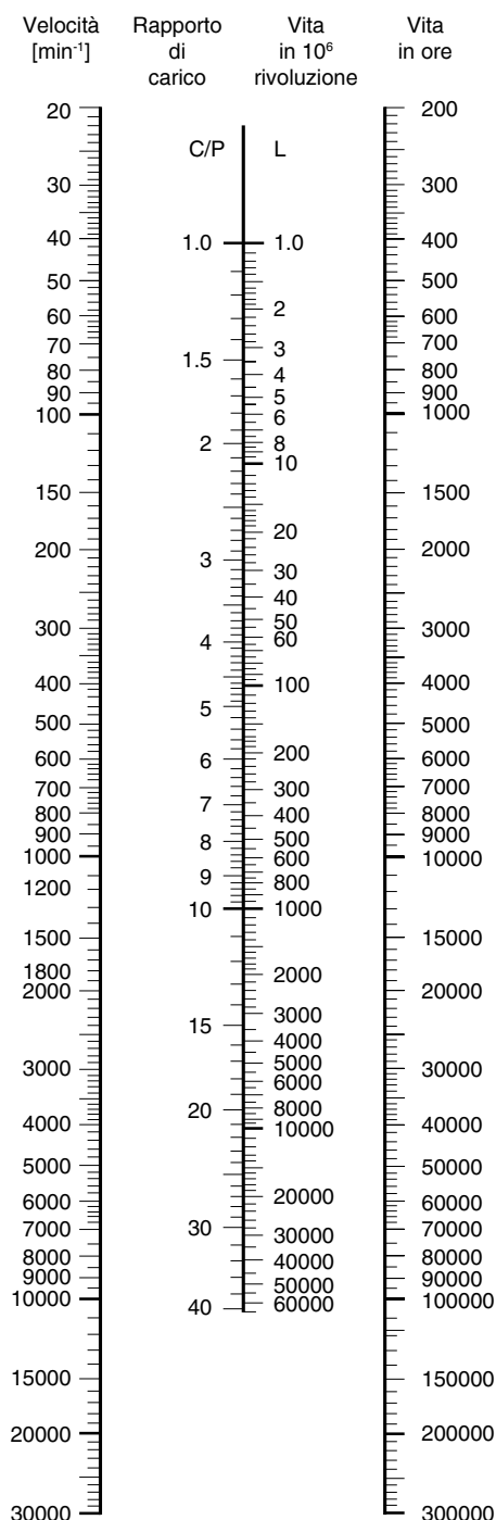
NORMOGRAFO (n-C/P-Lh)
